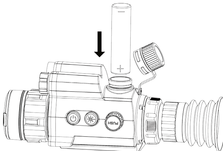
Figure 2-3 Installation de la batterie
