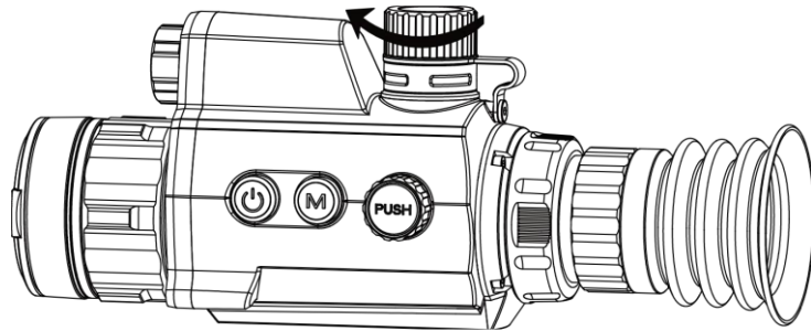
그림 2-4 배터리 커버 닫기
