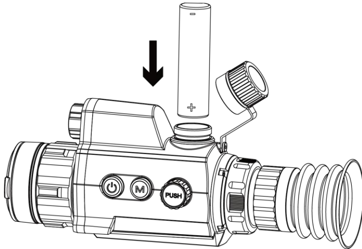
그림 2-3 배터리 설치
