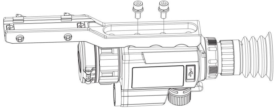
그림 2-6 나사 설치
