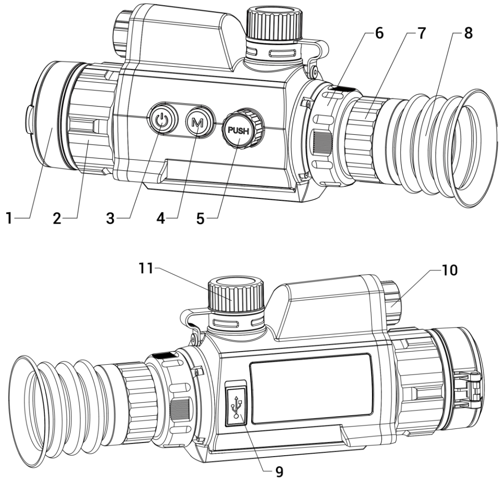
그림 1-1 장비의 외관
