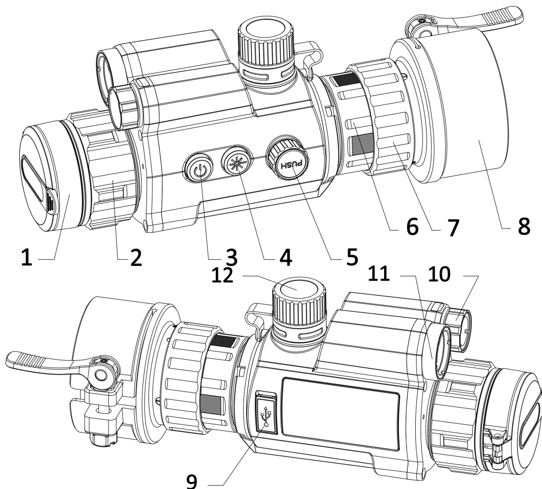
Rysunek 1-1 Wygląd urządzenia
