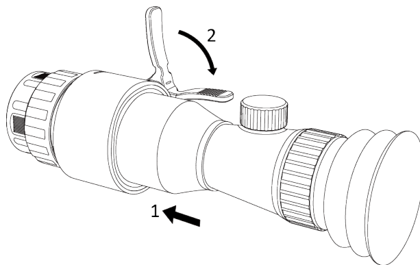
Rysunek 2-3 Instalowanie obiektywu optycznego
