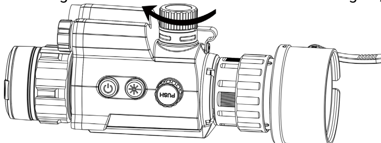
Rysunek 2-6 Zamykanie pokrywki baterii
