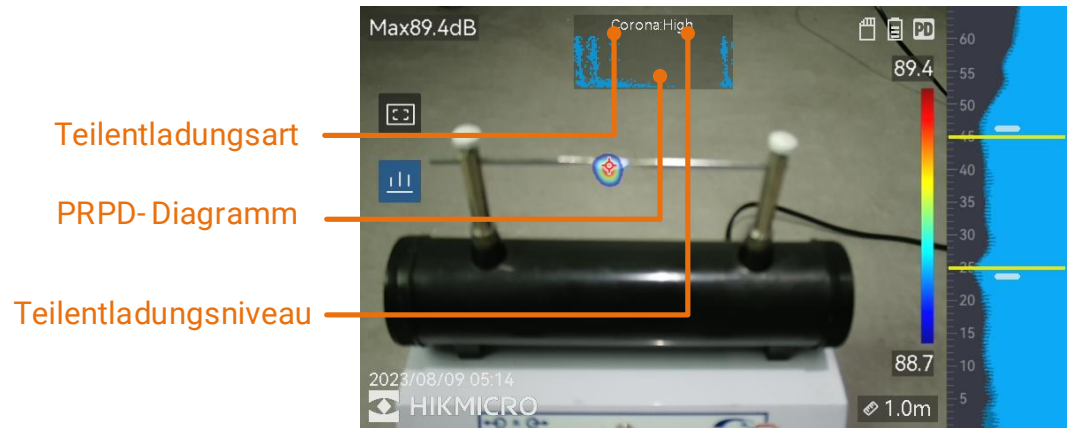
Abbildung 3-2 Teilentladungsanzeige
