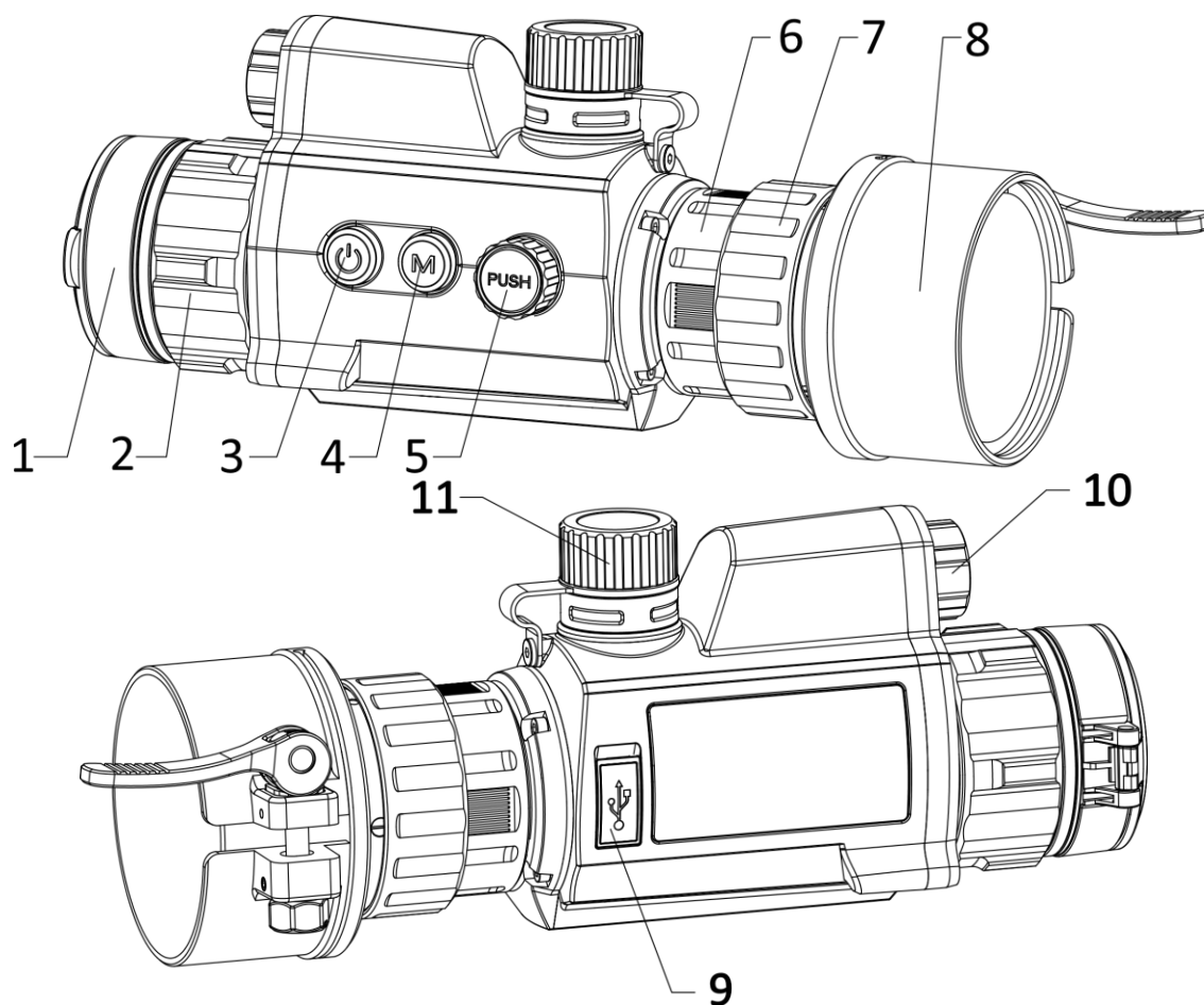
Figur 1-1 Enhetens utseende
