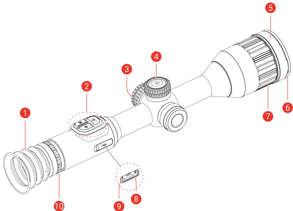
Abbildung 1-1 Aufbau
