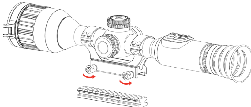
Abbildung 2-8 Schrauben lösen
