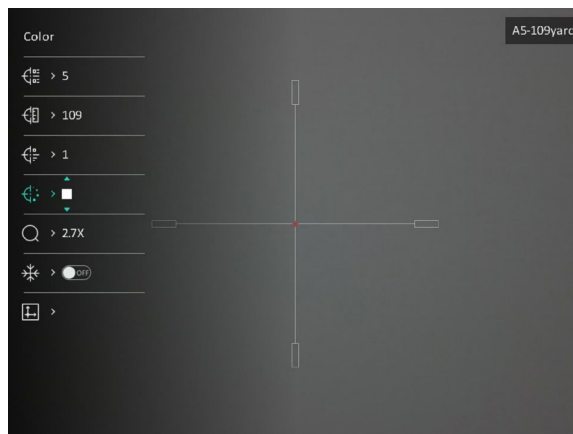
Figure 4-2 Correction du réticule
