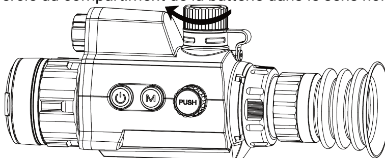
Figure 2-3 Installation de la batterie
