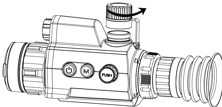
Figure 2-2 Ouverture du couvercle de la batterie
