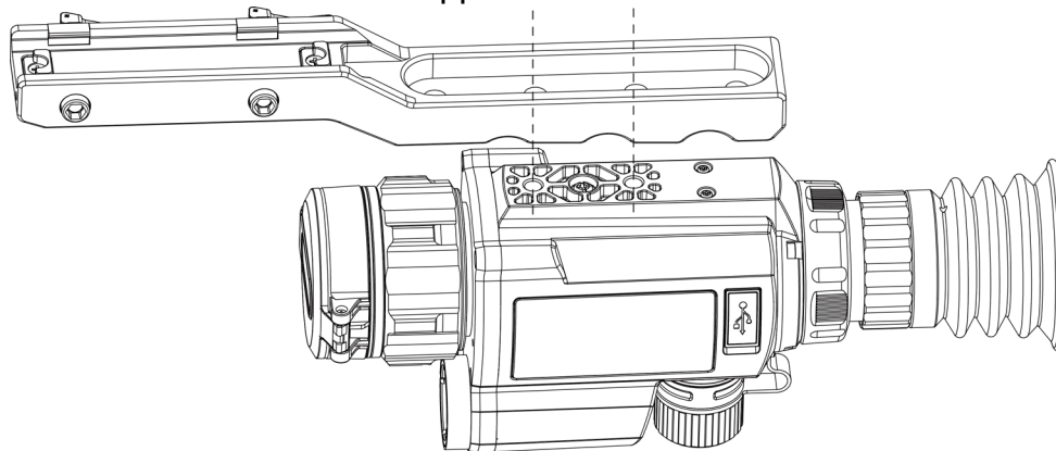
Figure 2-5 Alignement des trous d'installation
