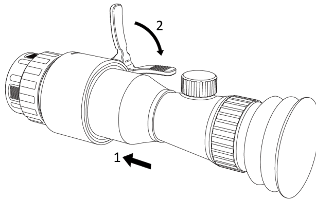
Abbildung 2-3 Tageslichtzielfernrohr montieren
