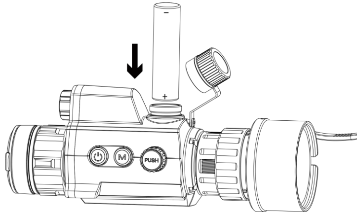
Abbildung 2-5 Akku einsetzen
