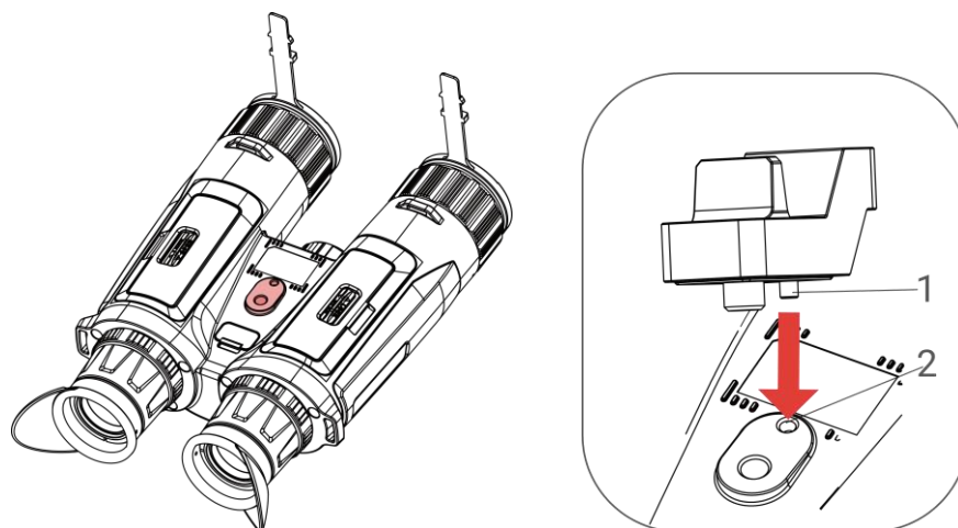
Figura 2-8 Inserção da coluna
