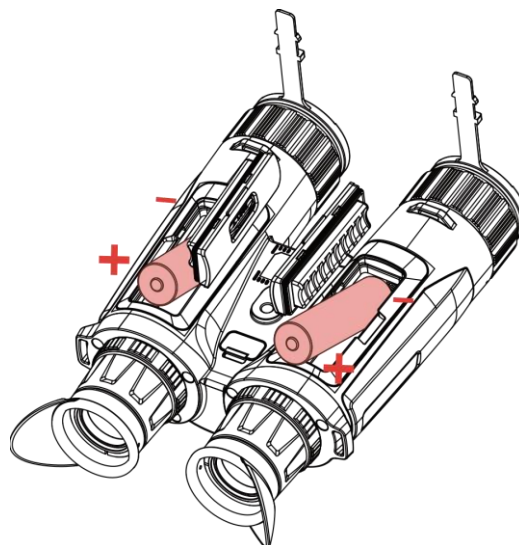
Figura 2-2 Instalação da bateria
