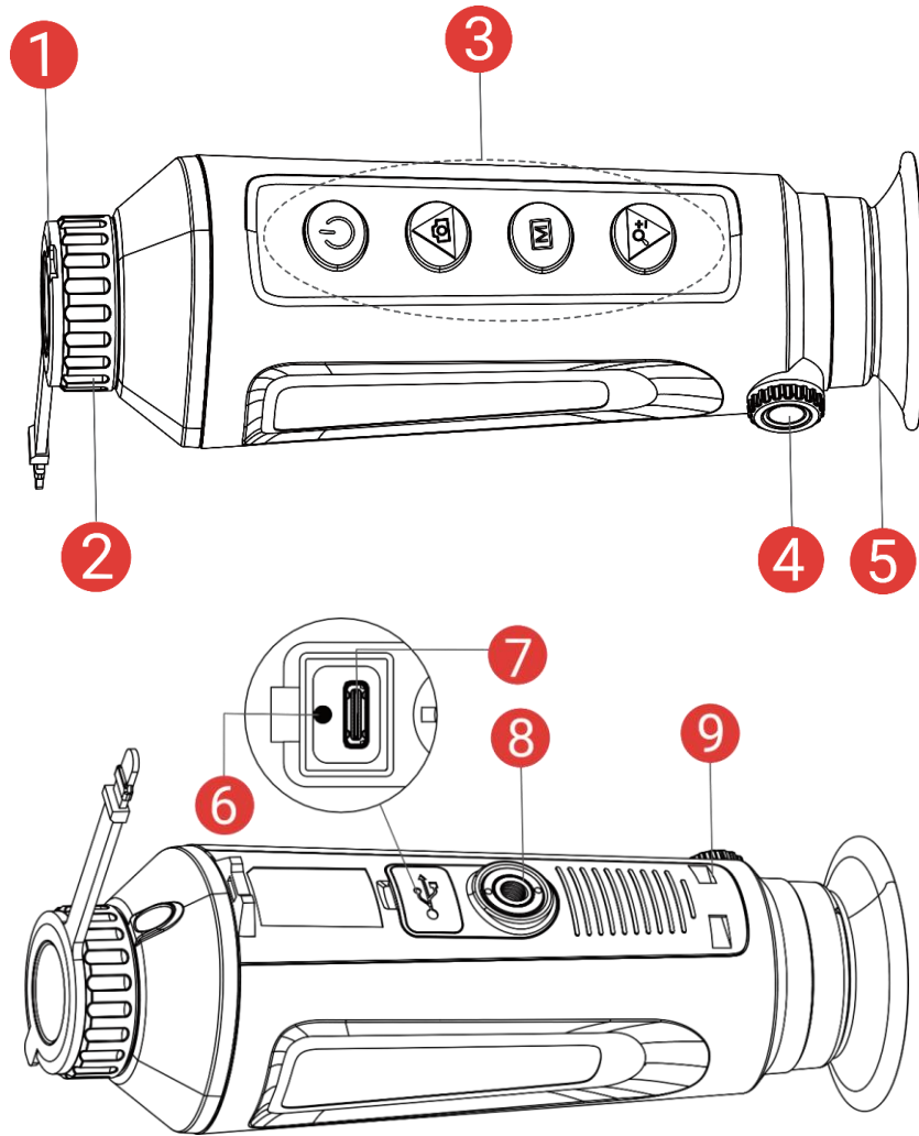
그림 1-1 외관
