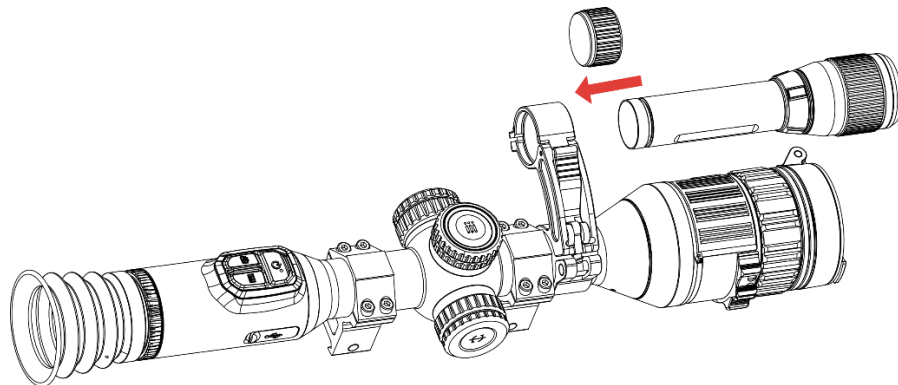
Rysunek 2-12 Mocowanie promiennika podczerwieni
