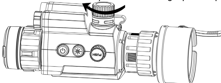
Figura 2-5 Instalação da bateria
