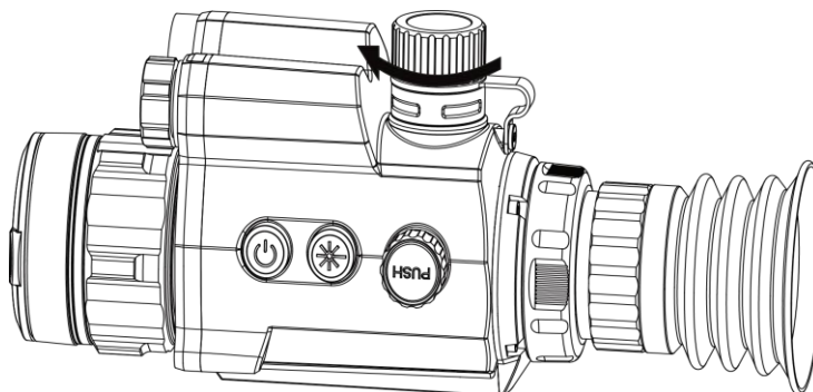
2-4. ábra: Az akkumulátorház fedelének lezárása
