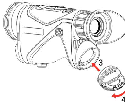
Рисунок 2-3 Закриття кришки
