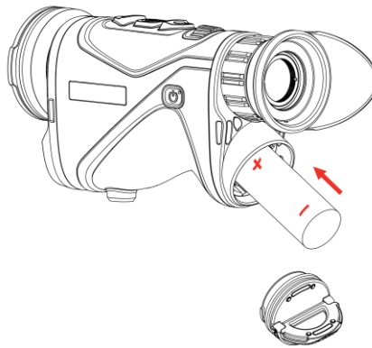
Рисунок 2-2 Уставте батарею
