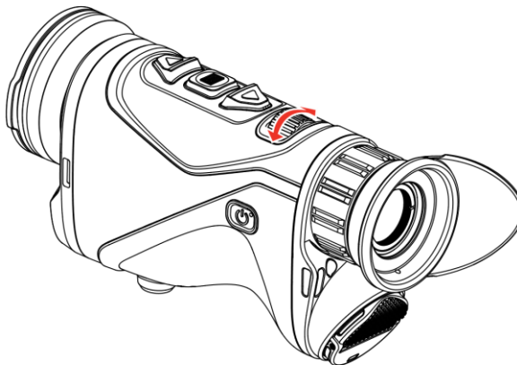
Рисунок 3-2 Регулювання фокуса
