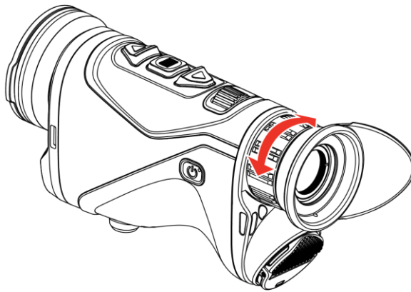
Рисунок 3-1 Регулювання діоптрій
