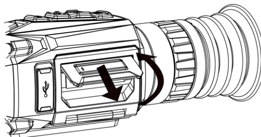
Abbildung 2-1 Entfernen der Abdeckung des Batteriefachs
