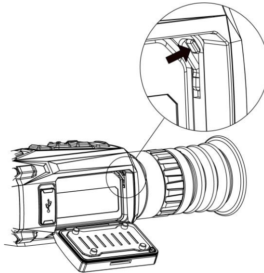
Abbildung 2-2 Entriegeln der Batterieverriegelung
