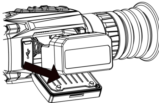
Abbildung 2-3 Einlegen der Batterie
