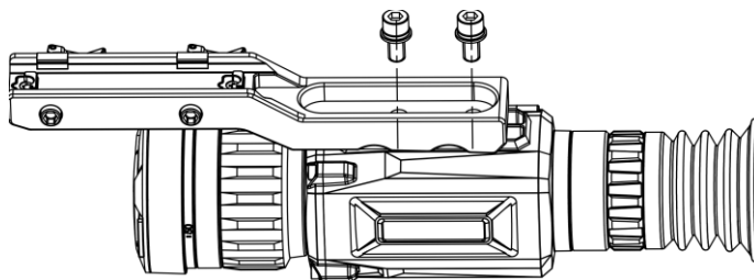
Abbildung 2-5 Schrauben einsetzen
