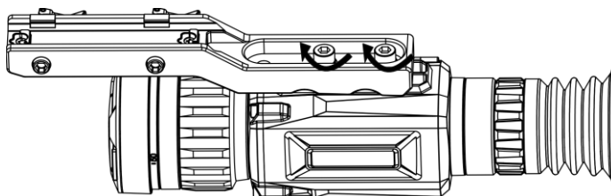
Abbildung 2-6 Gerät anschrauben
