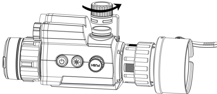
Figur 2-4 Åpne batteridekselet
