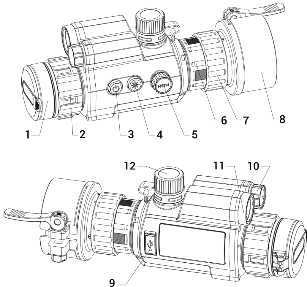
Figur 1-1 Enhetens utseende
