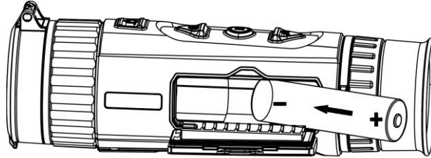
그림 2-3 배터리 설치
