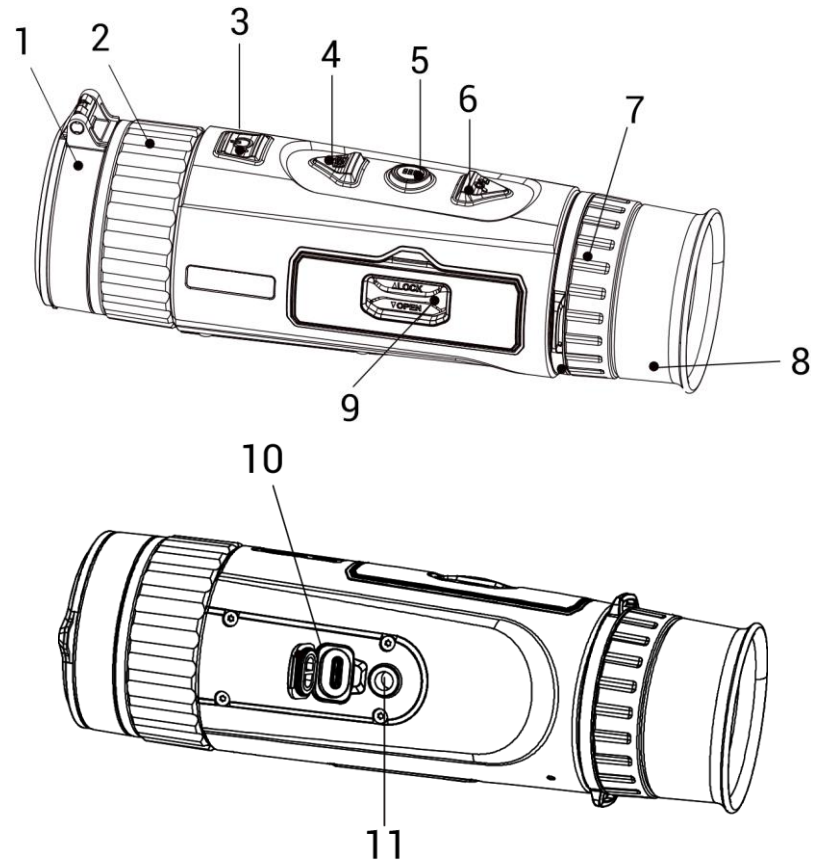
그림 1-1 외관
