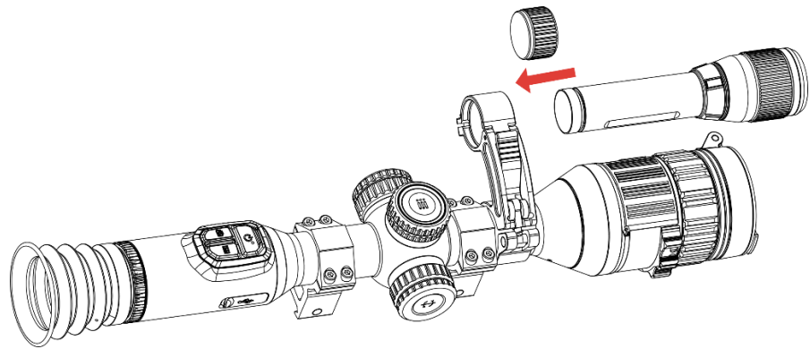
Figure 2-12 Mise en place de la torche IR
