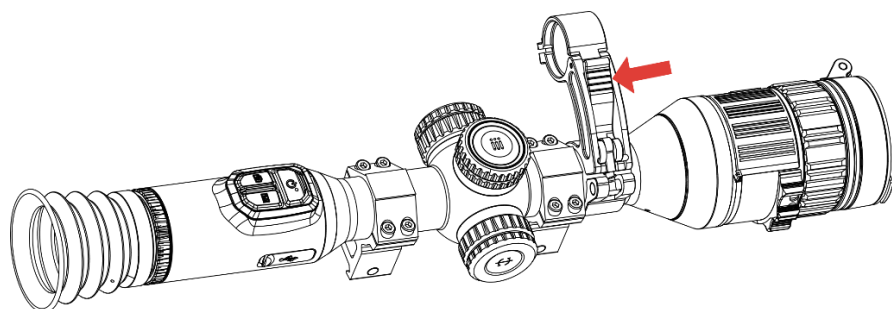
Figure 2-11 Blocage du levier
