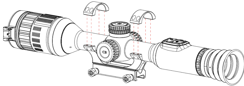
Figure 2-6 Installation de l'appareil dans la bague
