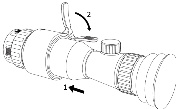
Figur 2-3 Montera dagsljuskikarsikte
