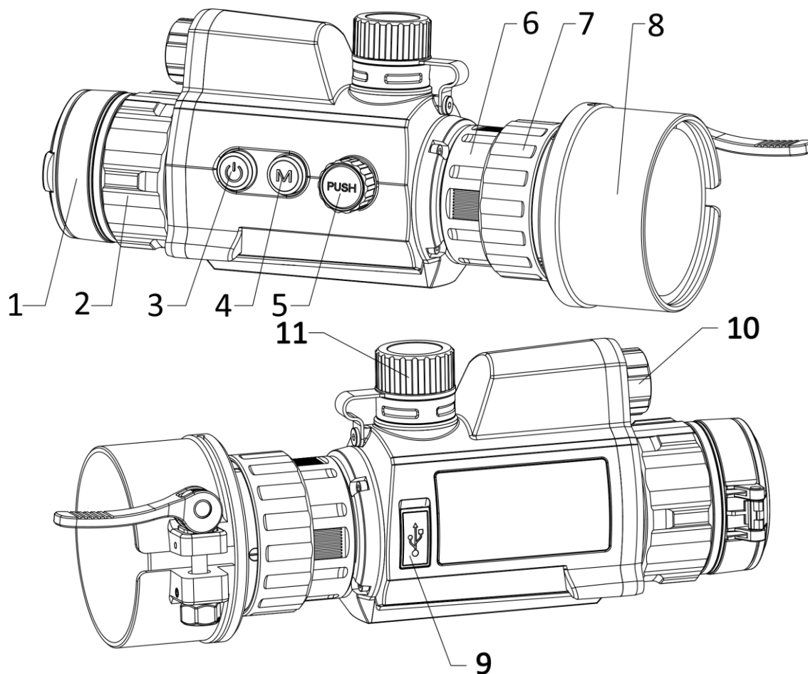
Figur 1-1 Enhetens utseende
