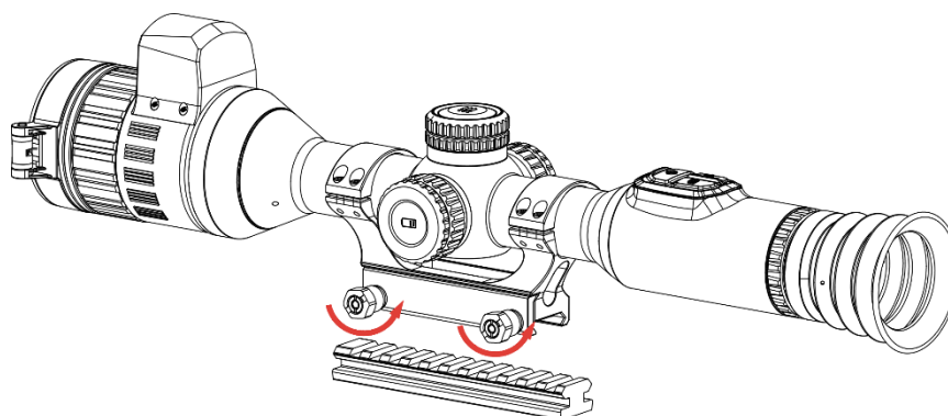
Figura 2-8 Aflojar los tornillos
