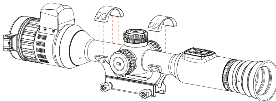
Figura 2-6 Colocar el dispositivo en el anillo
