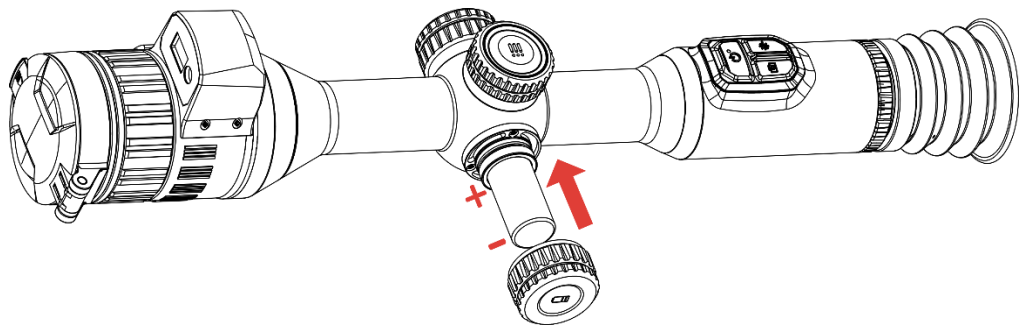
Figura 2-3 Insertar la batería
