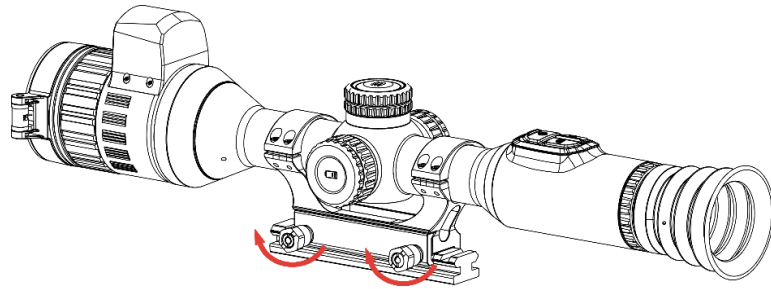
Figura 2-9 Apretar los tornillos
