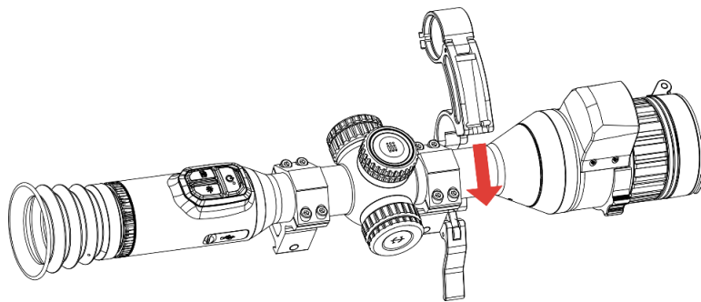
Figura 2-10 Abrir el soporte del iluminador IR
