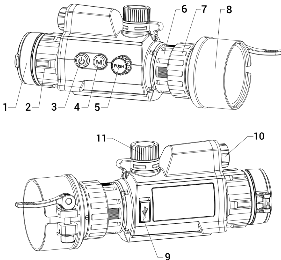
Rysunek 1-1 Elementy urządzenia
