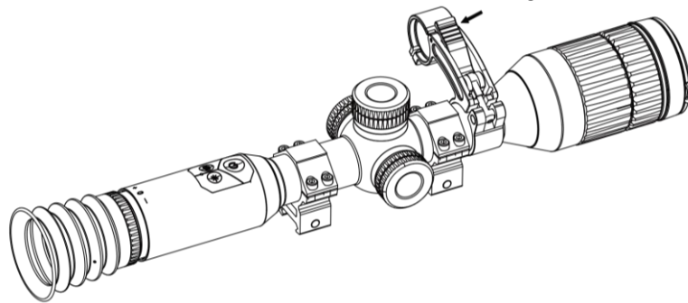
Abbildung 2-11 Hebel verriegeln
