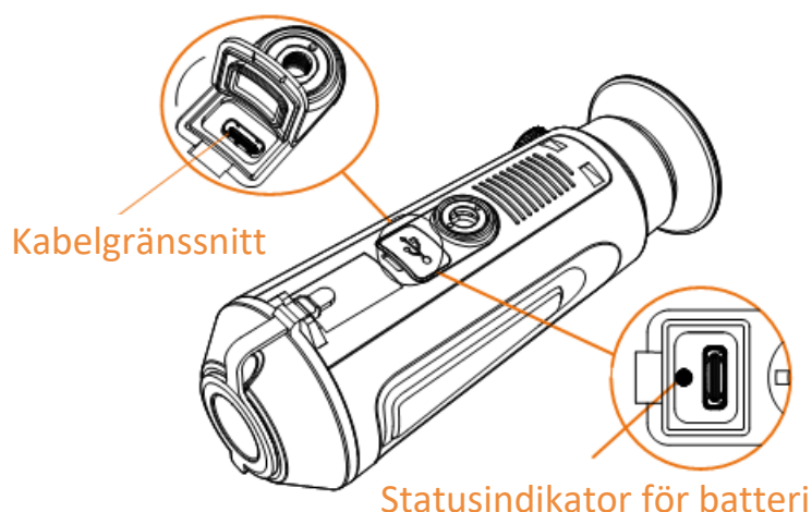
Figur 2-1 Kabelgränssnitt
