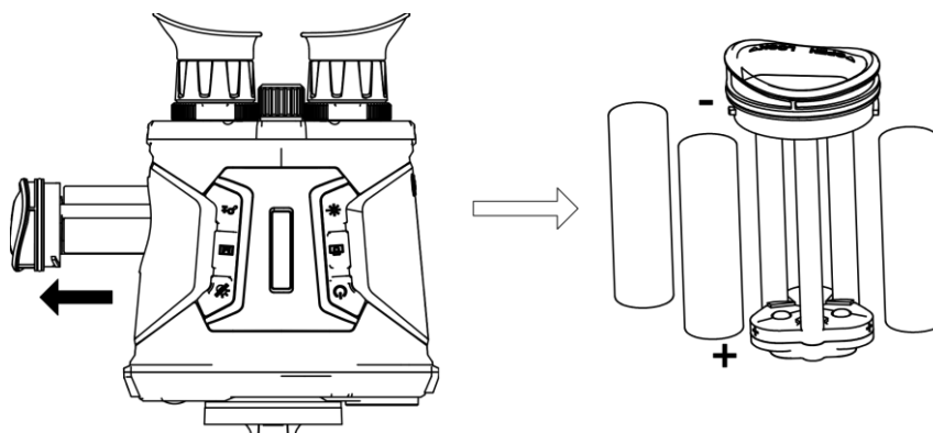
Figura 2-2 Installazione delle batterie
