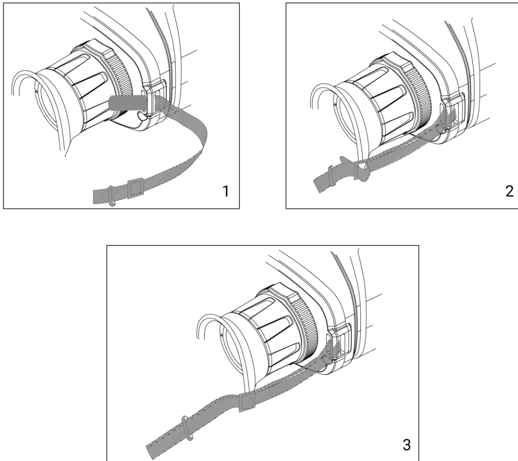
Figura 2-5 Montaggio della tracolla
