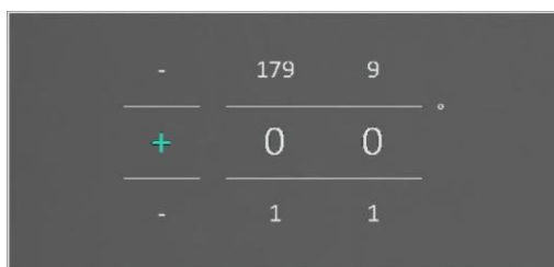
Figura 5-9 Correzione della declinazione magnetica
