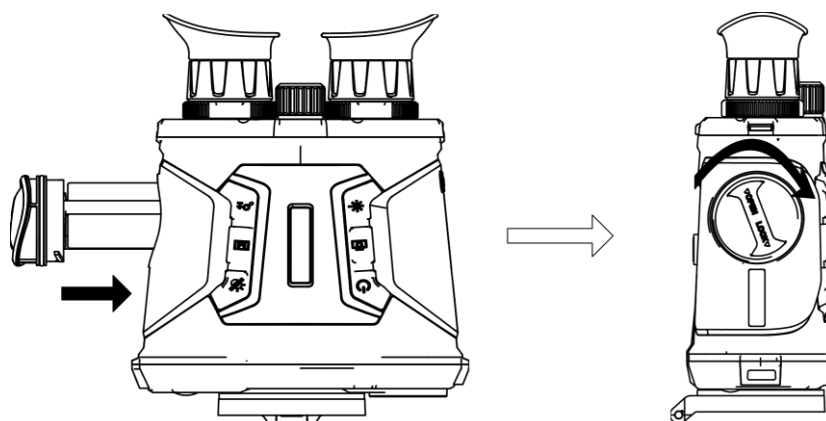
Figura 2-3 Installazione del vano batterie
