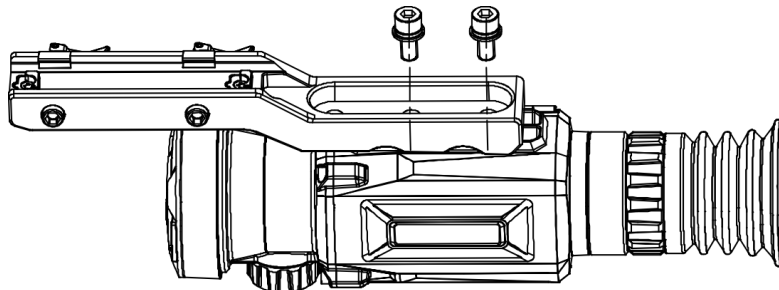
Abbildung 2-5 Schrauben einsetzen
