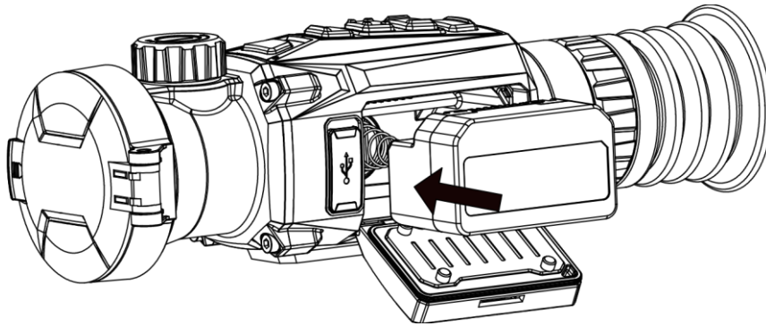
Abbildung 2-4 Einlegen der Batterie
