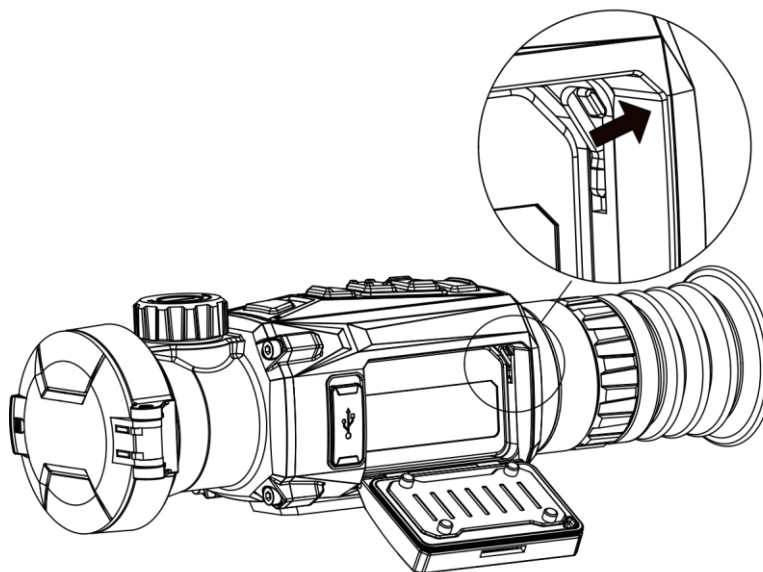
Abbildung 2-3 Entriegeln der Batterieverriegelung
