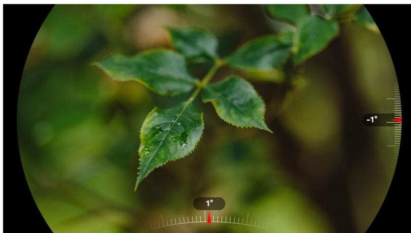
Figure 3-8 Échelle d'intervalles
