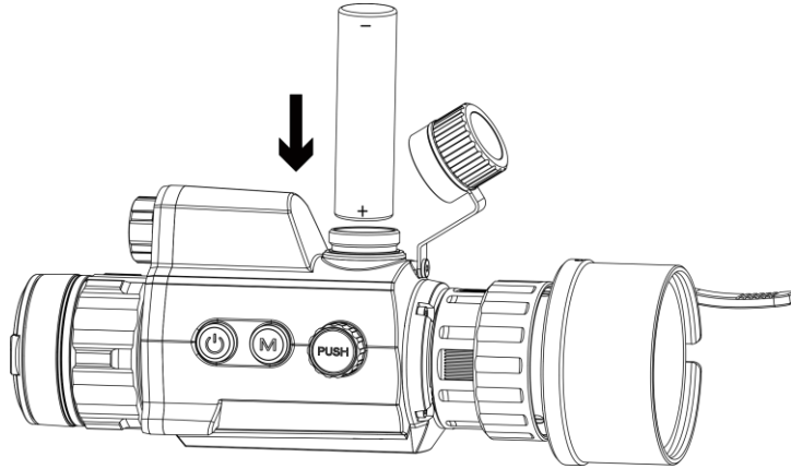
그림 2-5 배터리 설치
