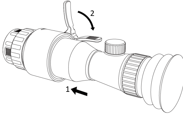
그림 2-3 일광 스코프 설치
