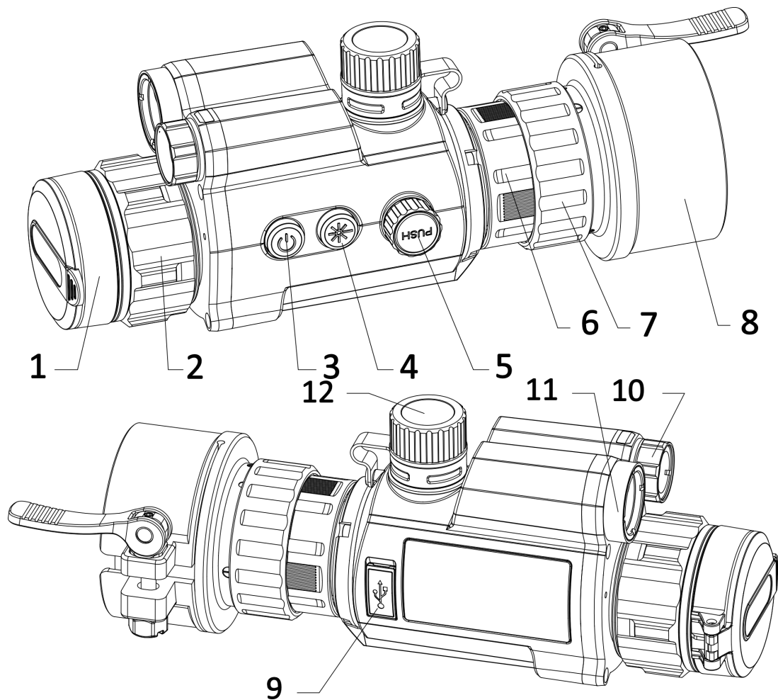
1-1 ábra Az eszköz megjelenése
