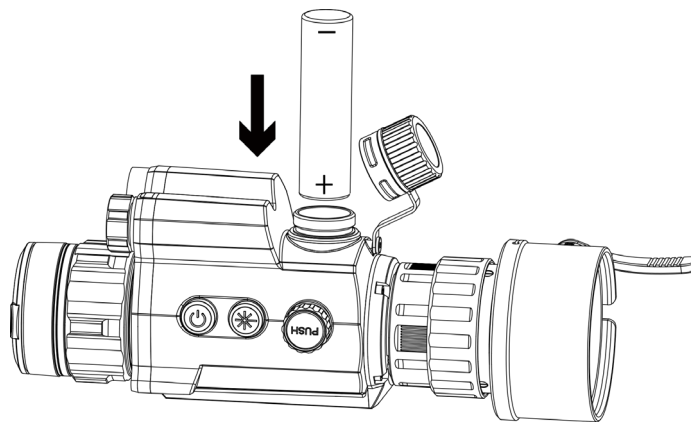
2-5 ábra Akkumulátor behelyezése
