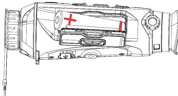
Figura 2-2 Insertar la pila
