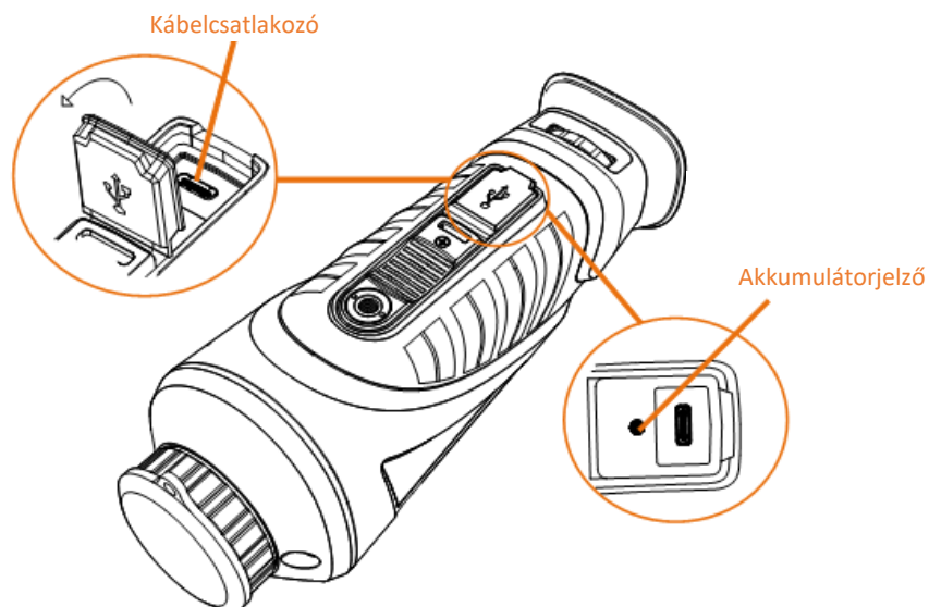
2-1. ábra Kábelcsatlakozó
