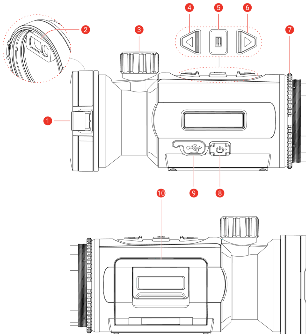
Obrázek 1-1 Vzhled
