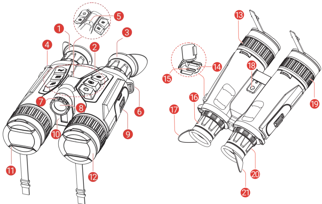
그림 1-1 외관
