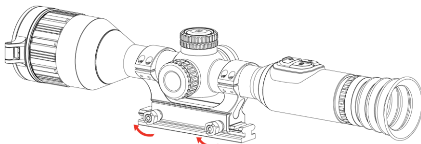
2-9 ábra Húzza meg a csavarokat
