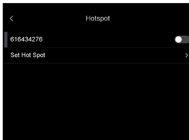
Abbildung 10-2 Hotspot festlegen
