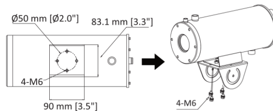
Figur 3-6 Installation af PT-beslagets overdel på kameraet
