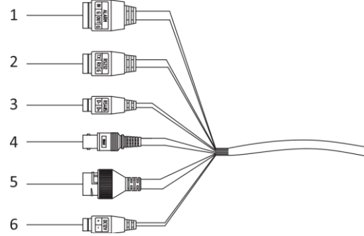
Şekil 2-2 Kamera Kabloları
