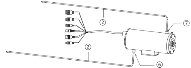
Gambar 3-10 Sambungan Pipa untuk Pendingin Air
