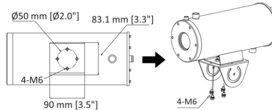
ပုံ 3-6 PT အဆက် ထိပ်ပိုင်းနှင့် ကင်မရာကို တပ်ဆင်ပါ
