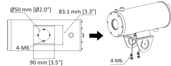
Afbeelding 3-6 De bovenkant van het PT-verbindingsstuk installeren op de camera
