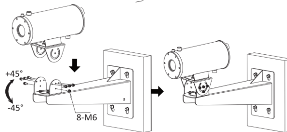
Figur 3-7 Justering af tiltvinkel
