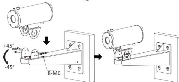
Рисунок 3-7. Відрегулюйте кут нахилу
