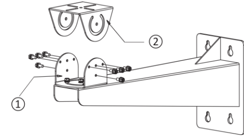
図 3-3 PT ジョイントの分解
