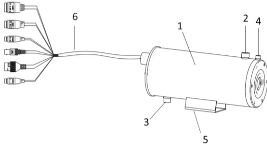
ပုံ 2-1 ပုံပန်း သွင်ပြင်
