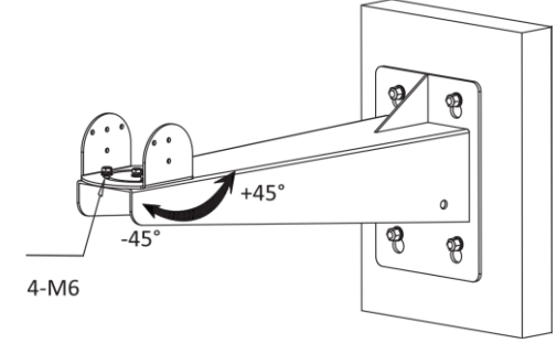
Şekil 3-5 Kaydırma Açısını Ayarlayın
