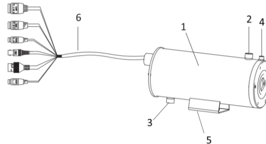
그림 2-1 외관
