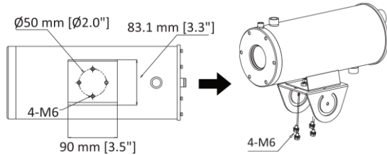
Figura 3-6 Instalați partea superioară a articulației PT pe cameră
