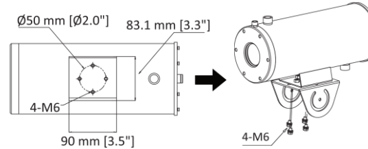
Abbildung 3-6 Oberseite des PT-Gelenks mit Kamera installieren
