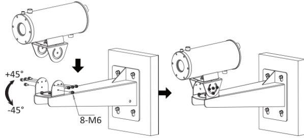
Şekil 3-7 Eğim Açısını Ayarlayın
