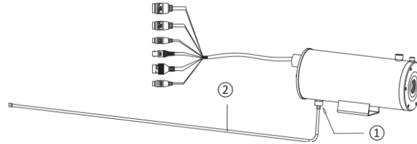
Figure 3-8 Raccordement du tuyau pour le refroidissement par air
