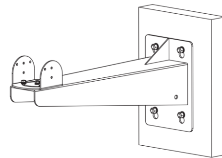
Figura 3-4 Instalarea suportului
