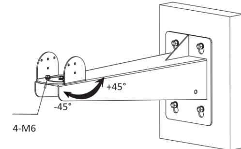
Figure 3-5 Réglage de l'angle de panoramique
