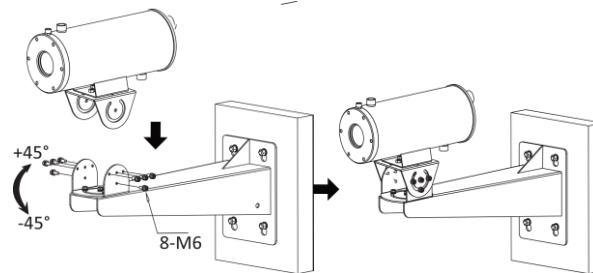
Imagen 3-7 Ajustar el ángulo de inclinación
