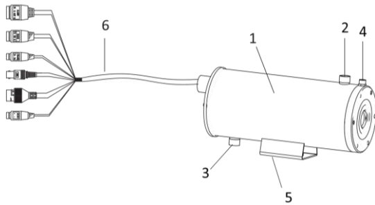
Figura 2-1 Aspect
