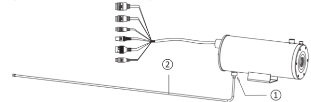
Abbildung 3-8 Rohranschluss für Luftkühlung
