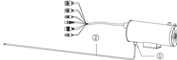
3-8 ábra Léghűtő cső csatlakoztatása
