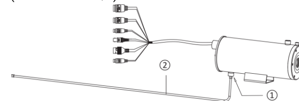
Imagen 3-8 Conexión del tubo para el enfriamiento por aire
