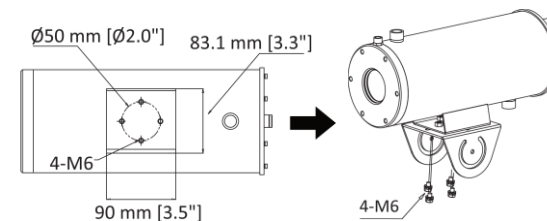
Рисунок 3-6. Присоединение верх шарнирного соединения с камерой
