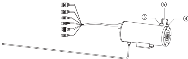
그림 3-9 방진 설치
