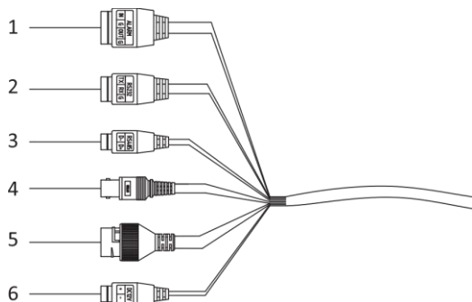
Obrázek 2-2 Kabely kamery
