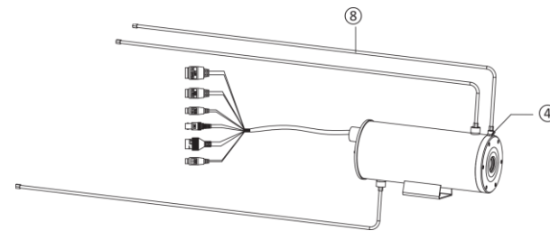
Obrázek 3-11 Instalace odstranění prachu
