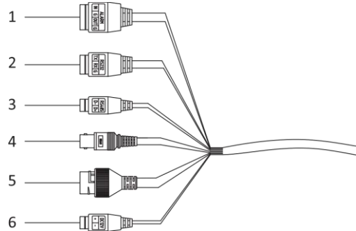
Figura 2-2 Cablurile camerei
