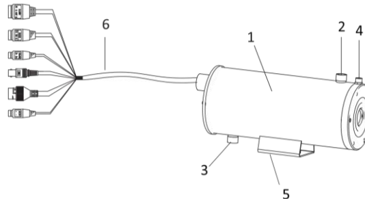
Figura 2-1 Aspeto
