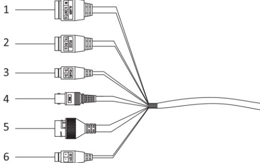
Imagen 2-2 Cables de la cámara
