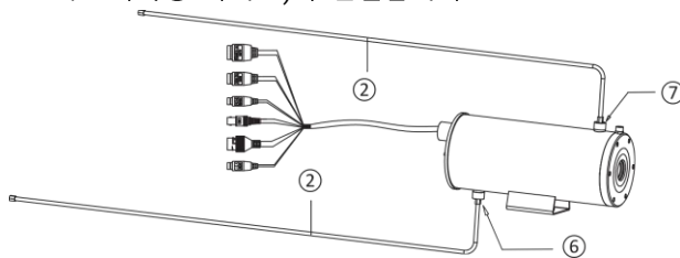
그림 3-10 수랭식 파이프 연결
