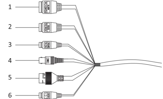
Abbildung 2-2 Kabel der Kamera
