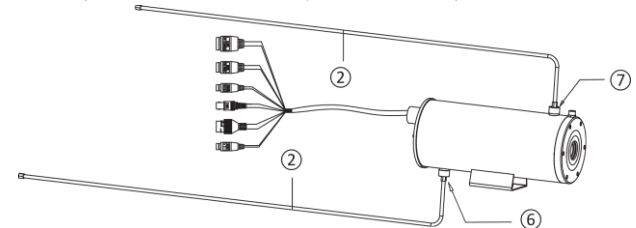
Figura 3-10 Conexiunea conductei pentru răcirea cu apă
