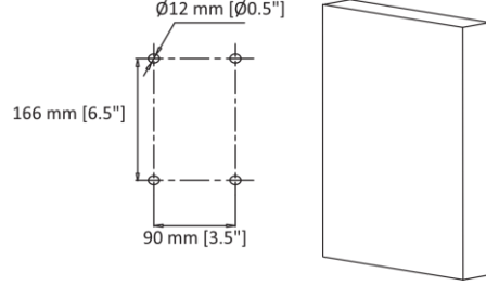
Şekil 3-1 Duvara Delikler Delin
