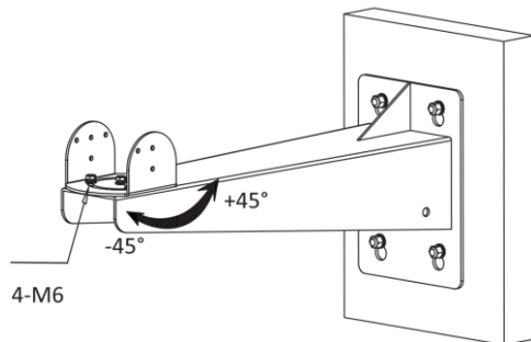
Figur 3-5 Justering af panoreringsvinkel
