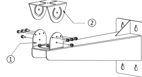
Рисунок 3-3. Розберіть поворотно-нахильний кронштейн
