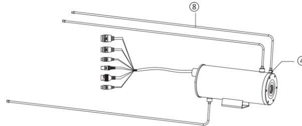
Abbildung 3-11 Entstaubende Installation
