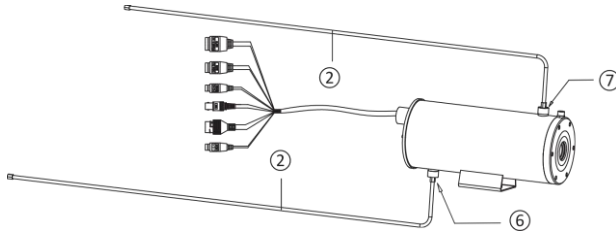
Figure 3-10 Raccordement du tuyau pour le refroidissement par eau
