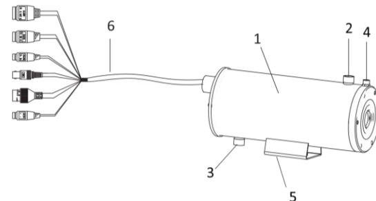
Рисунок 2-1. Внешний вид
