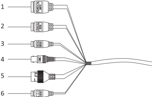
圖 2-2 攝影機纜線
