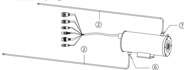
Figura 3-10 Collegamento del tubo per il raffreddamento ad acqua
