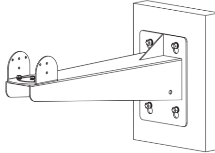
Şekil 3-4 Braketi Takın
