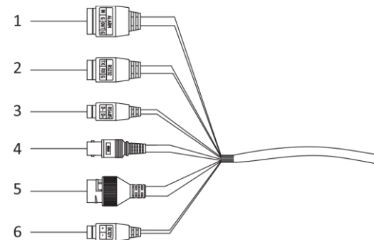
Рисунок 2-2. Кабелі камери
