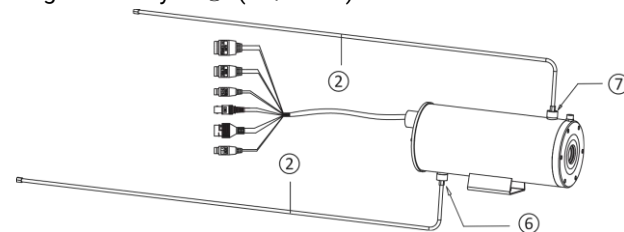
Rysunek 3-8 Podłączanie przewodu doprowadzającego powietrze chłodzące
