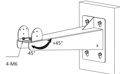
3-5 ábra Állítsa be a pásztázási szöget
