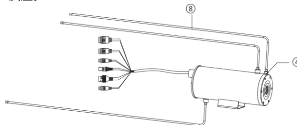
圖 3-11 除塵安裝
