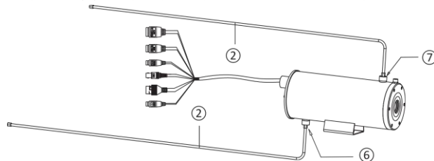
圖 3-10 水冷管路連接
