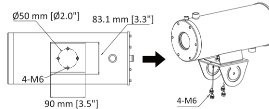
Figura 3-6 Instale o topo da junta PT com a câmara
