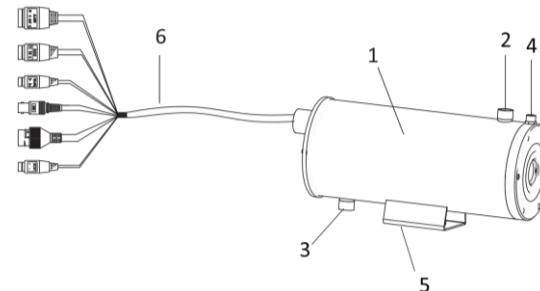
Afbeelding 2-1 Uiterlijk
