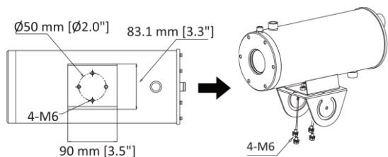
Rysunek 3-6 Mocowanie górnej części uchwytu uchylnego do kamery
