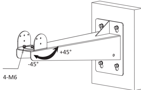
Abbildung 3-5 Schwenkwinkel anpassen
