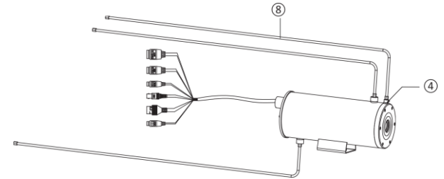
Figura 3-11 Instalação de despoejamento
