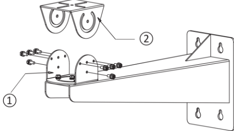
Afbeelding 3-3 Het PT-verbindingsstuk demonteren
