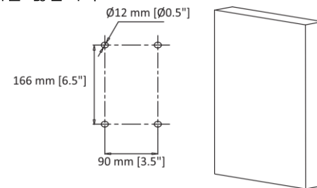
그림 3-1 벽면 드릴 구멍
