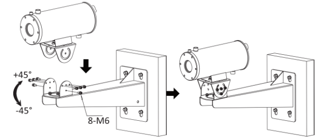
Afbeelding 3-7 De kantelhoek aanpassen
