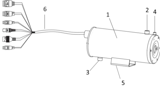
Şekil 2-1 Görünüm
