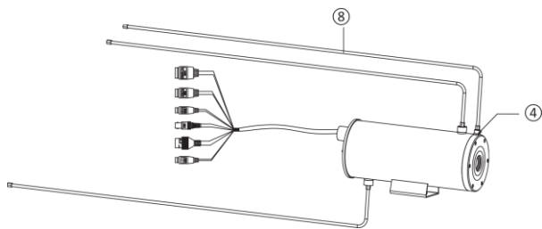
Рисунок 3-11. Установка системы удаления пыли
