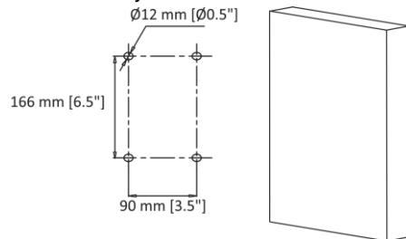
Obrázok 3-1 Vyrývajte do steny otvory
