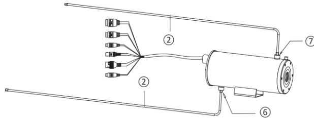
Abbildung 3-10 Rohranschluss für Wasserkühlung
