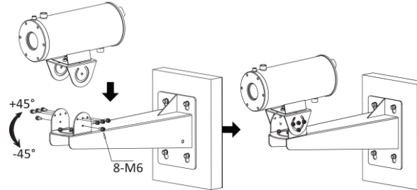
Abbildung 3-7 Neigungswinkel anpassen
