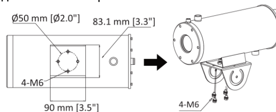
Рисунок 3-6. Установіть верхню частину поворотно-нахильного кронштейна на камеру
