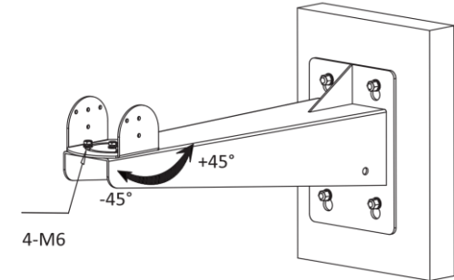
Gambar 3-5 Atur Sudut Pelimbangan
