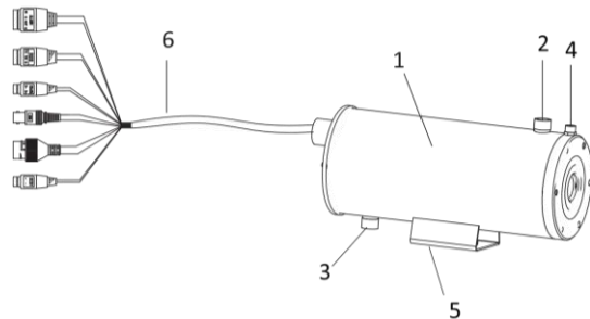
Рисунок 2-1. Зовнішній вигляд
