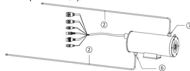
Рисунок 3-10. Присоединение труб для водяного охлаждения
