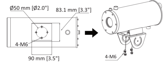
Şekil 3-6 PT Bağlantısının Üst Kısımını Kamerayla Birlikte Takın
