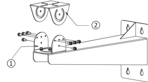
Abbildung 3-3 PT-Gelenk demontieren
