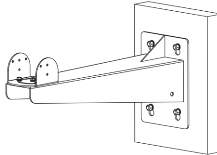
Afbeelding 3-4 De beugel installeren
