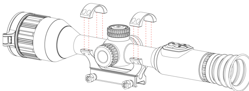
Figure 2-6 Installation de l'appareil dans la bague
