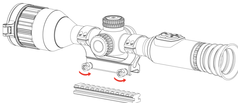
Figure 2-8 Desserrage des vis
