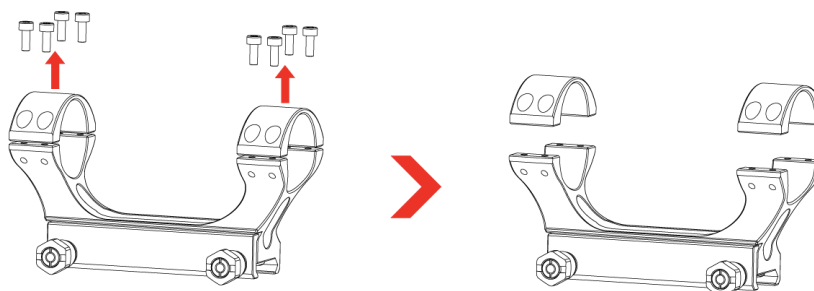
Figure 2-5 Dévissage du haut de la bague
