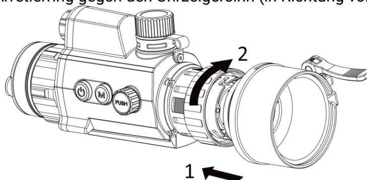
Abbildung 2-2 Adapter installieren
