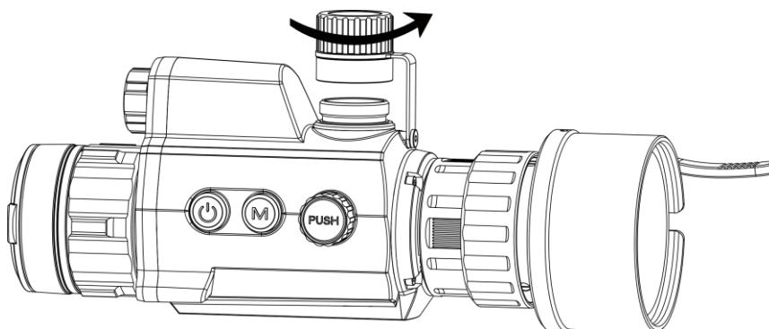
Abbildung 2-3 Akkufachdeckel öffnen
