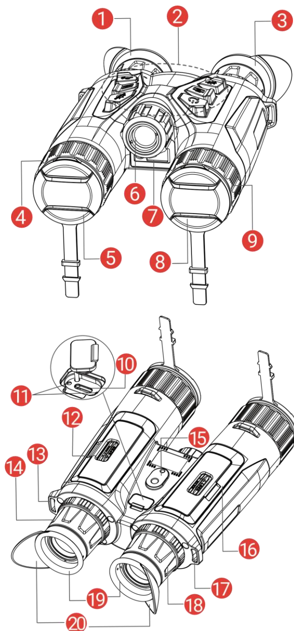
図 1-1 外観
