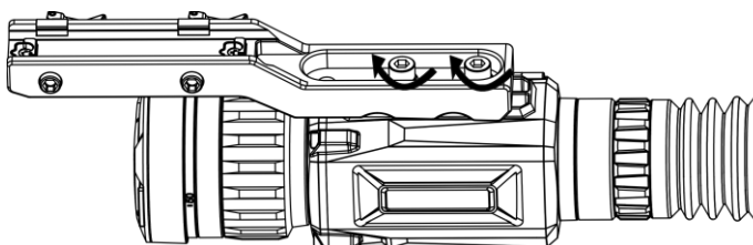
Figur 2-6 Sikre enheten
