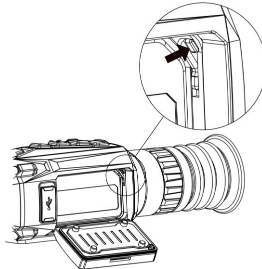
Figur 2-2 Løsne batterilåsen
