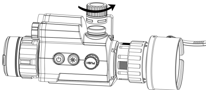
Afbeelding 2-3 Open batterijklepje
