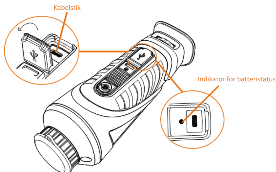
Figur 2-1 Kabelstik
