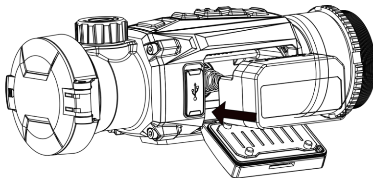
Obrázok 2-3 Vloženie batérie
