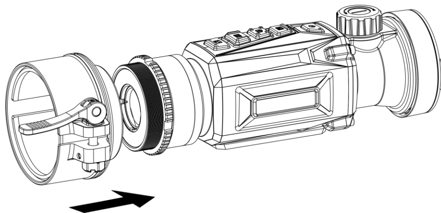
Obrázok 2-5 Inštalácia adaptéra
