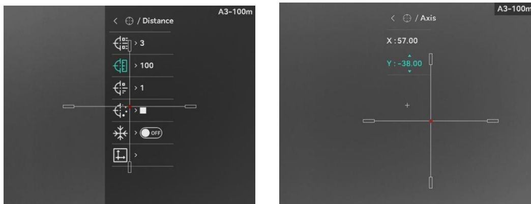
Rysunek 2-11 Zerowanie
