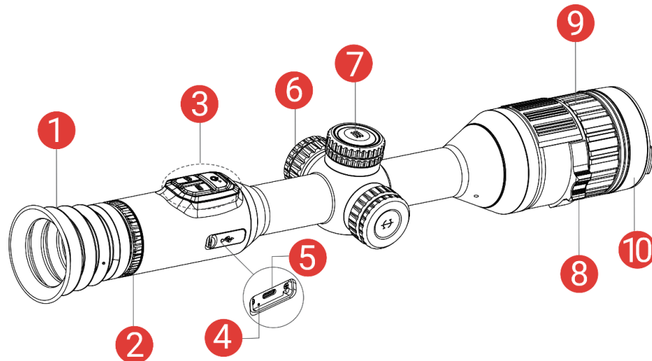
Abbildung 1-1 Aufbau
