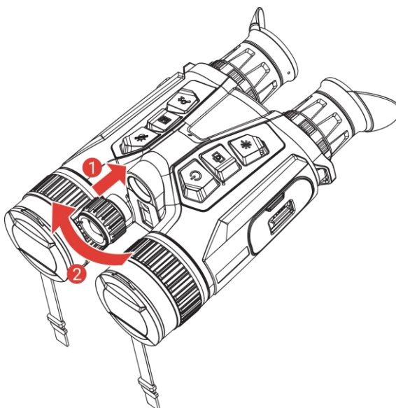
Figura 2-8 Montar o iluminador
