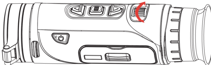
3-2 pav. Fokusavimo reguliavimas
