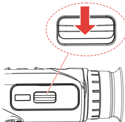
2-1 pav. Atidarykite akumulatoriaus skyriaus dangtelį.
