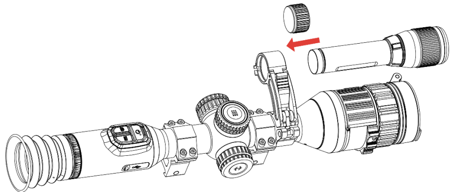
Abbildung 2-12 Befestigen der IR-Taschenlampe
