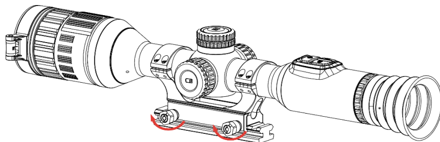
Abbildung 2-9 Festziehen der Schrauben
