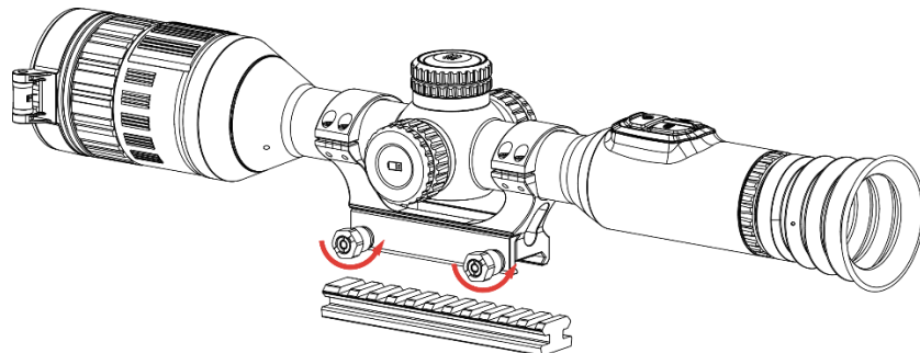
Abbildung 2-8 Schrauben lösen
