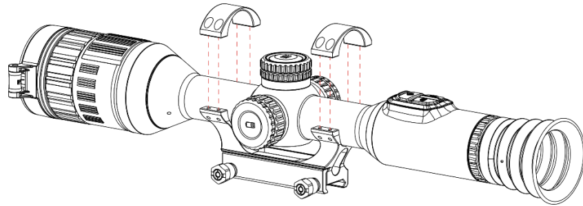
Abbildung 2-6 Legen Sie das Gerät in den Ring
