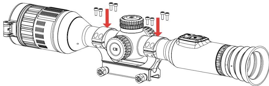
Abbildung 2-7 Festziehen der Schrauben
