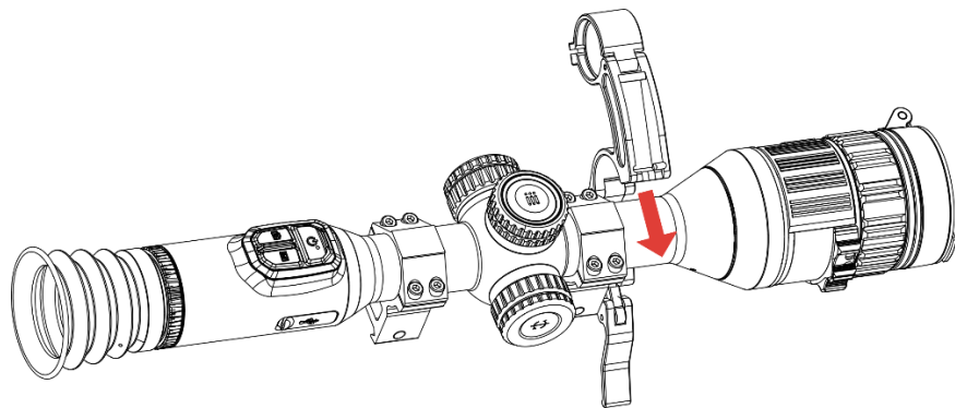
Abbildung 2-10 Öffnen der Halterung der IR-Lampe
