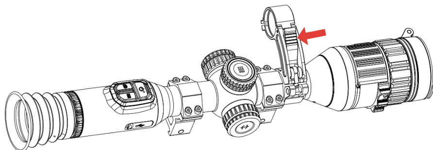
Abbildung 2-11 Verriegeln des Hebels
