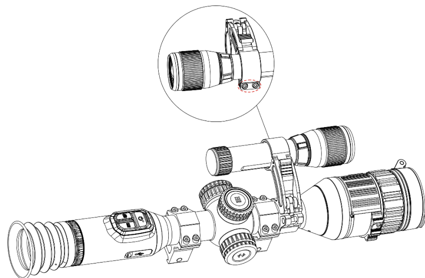
Abbildung 2-13 Fixieren der IR-Lampe
