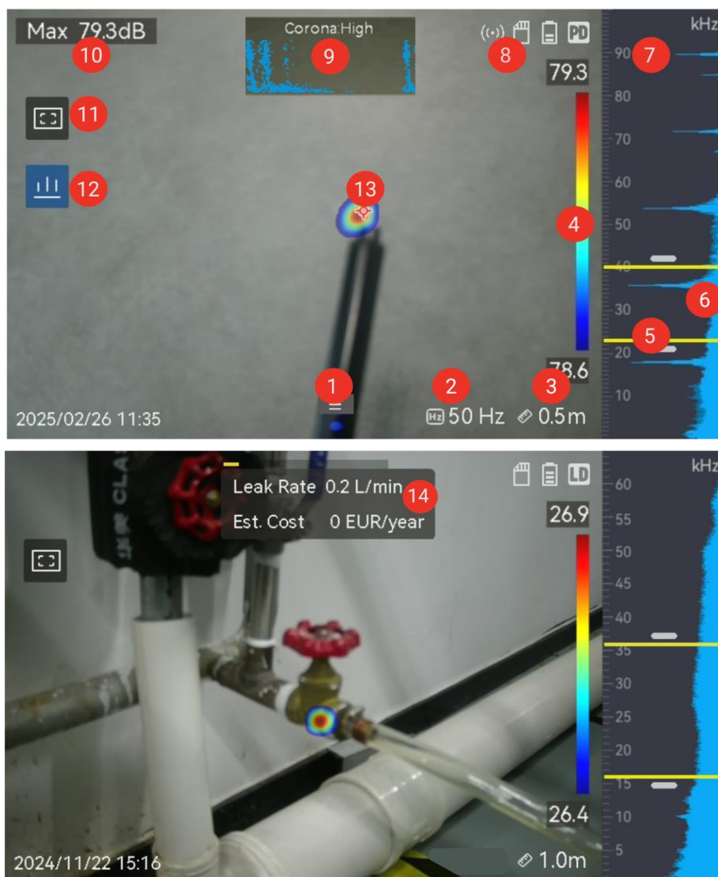
図 2-10 音響画像モードのライブビューインターフェイス
