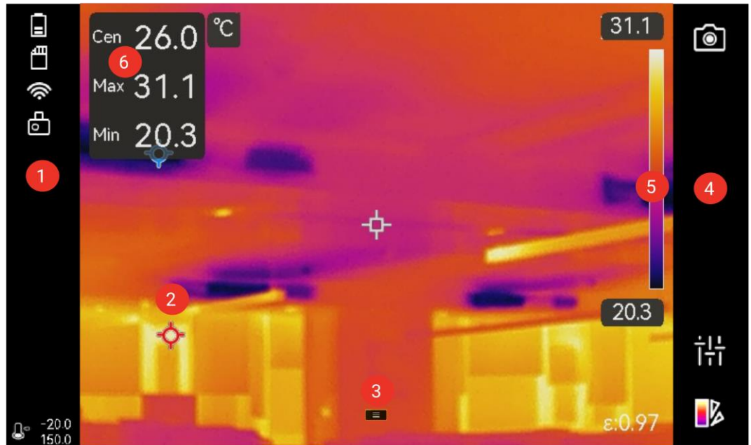
図 2-11 熱画像モードのライブビューインターフェイス
