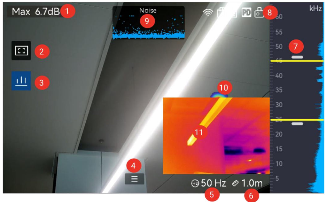
図 2-12 PIP 画像モードのライブビューインターフェイス
