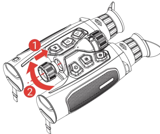
Abbildung 2-6 Montieren Sie den Strahler
