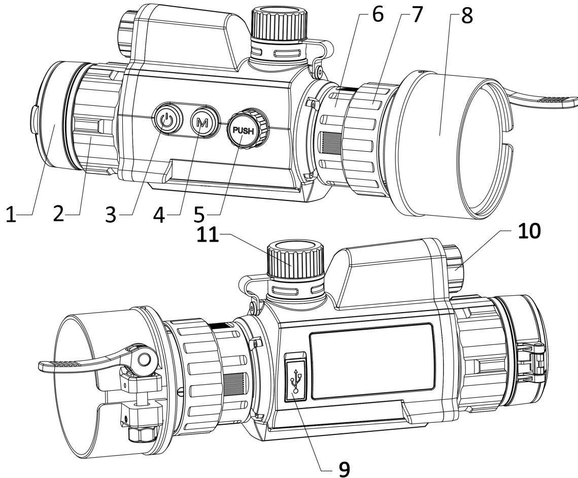
1-1 ábra Az eszköz megjelenése
