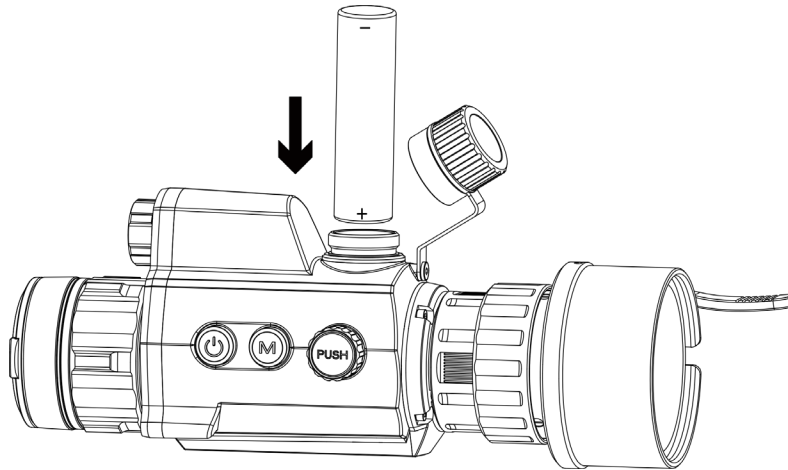
2-5 ábra Akkumulátor behelyezése
