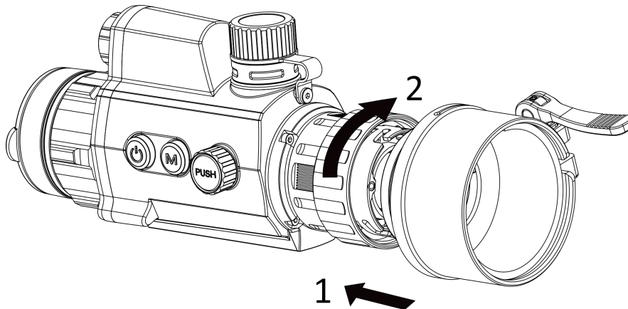
2-2 ábra Az adapter beszerelése
